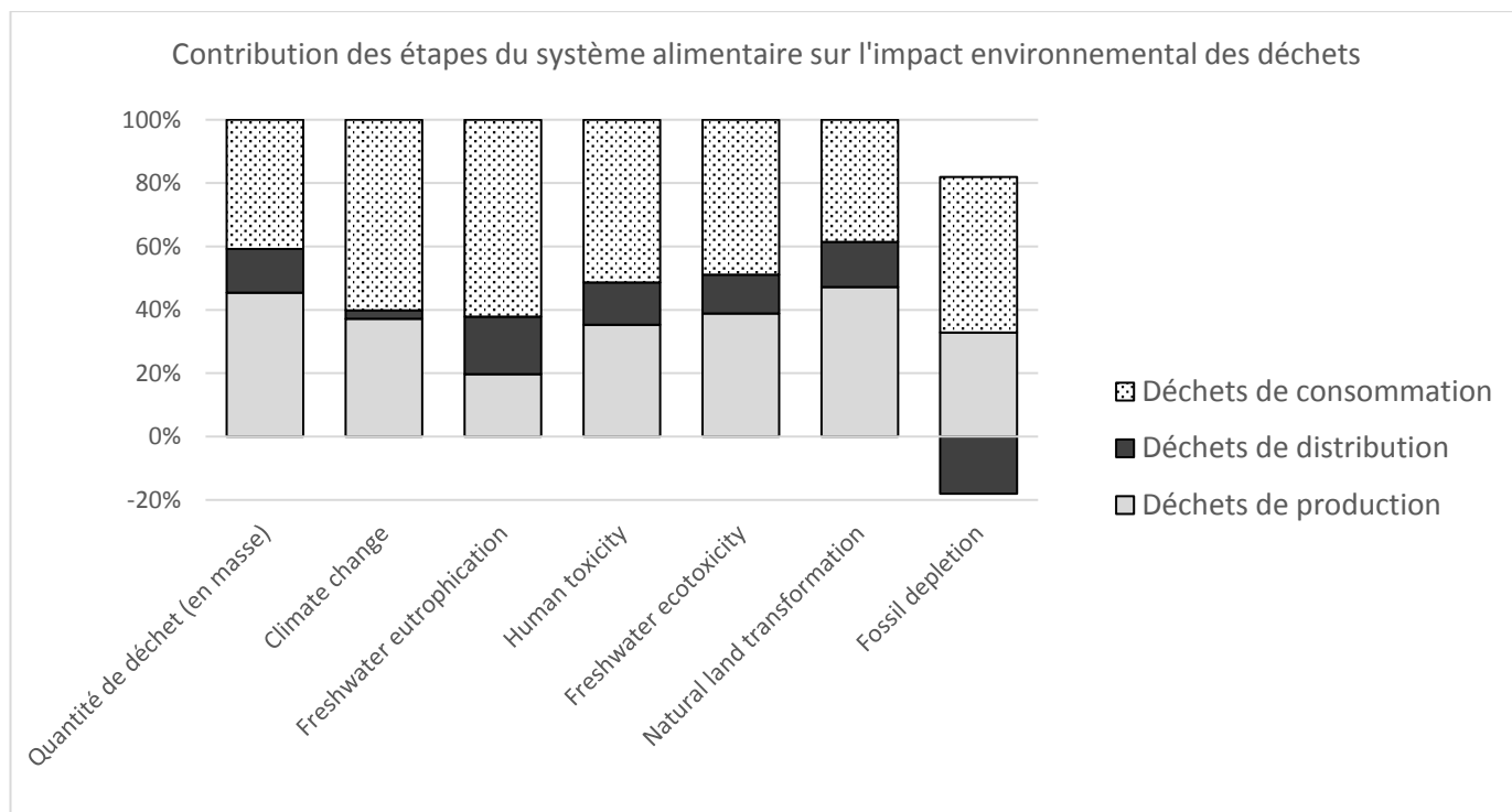
Figure 30: Contribution des étapes du système alimentaire sur l'impact environnemental des déchets (fin de vie incluse)
