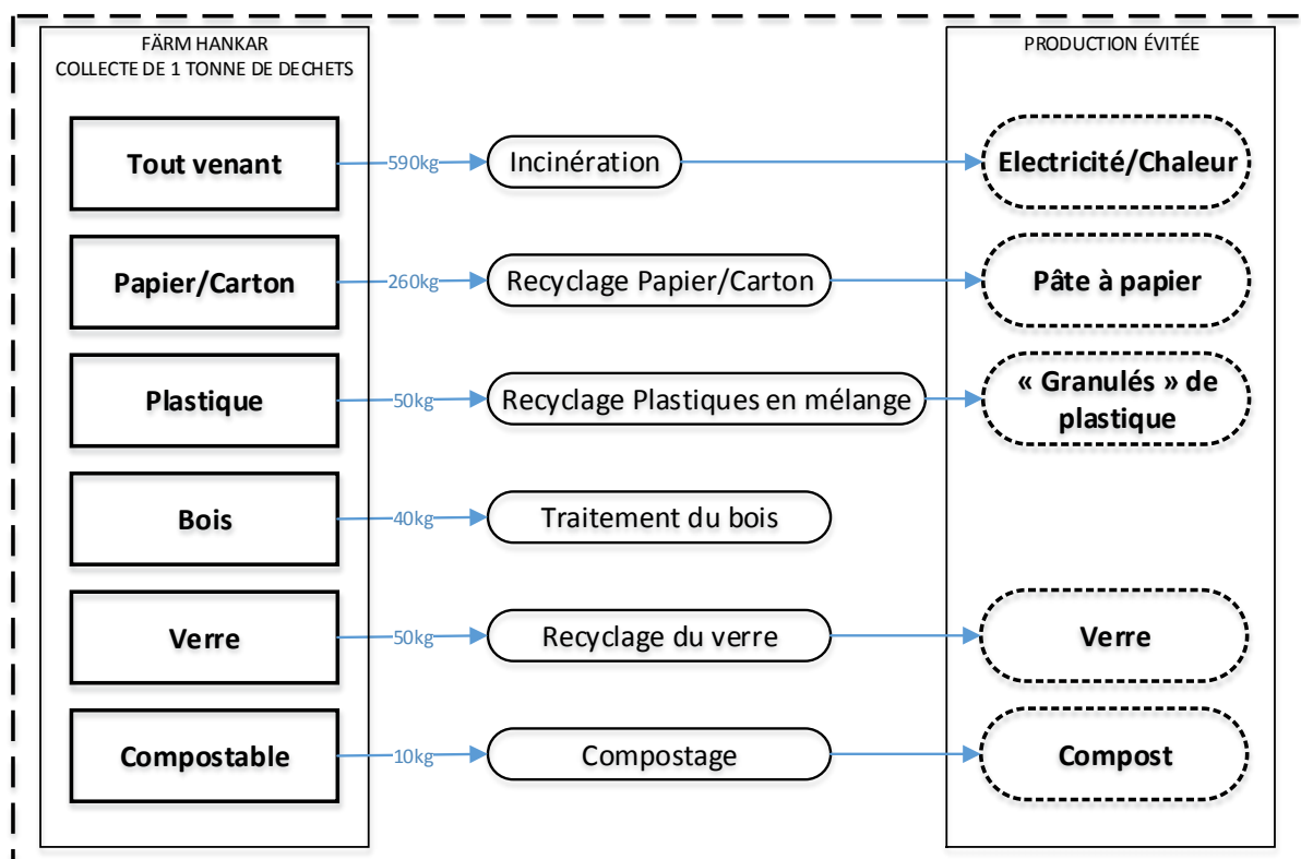
Figure 21 : Limites du système - ACV déchets Färm
