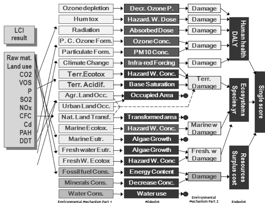
Figure 12 : Relation entre l'inventaire de l'ACV (gauche), les indicateurs midpoint (milieu) et les indicateurs endpoint (droite).
