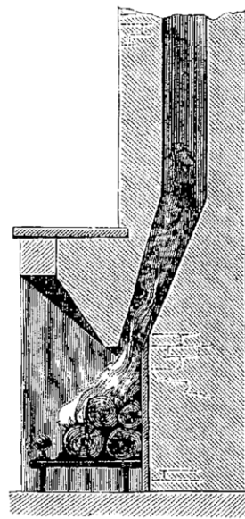
fig. 4 : Représentation de la cheminée Rudolf
