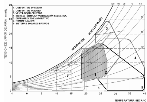
fig. 26 : Zones de confort étendu de Givoni
