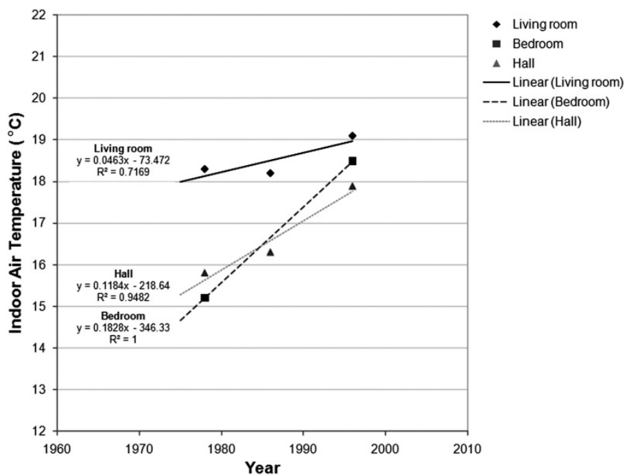
fig. 23 : Tendances des températures diurnes moyennes hivernales de l'air intérieur basées sur des enquêtes nationales auprès des ménages au Royaume-Uni (1978-1996)
