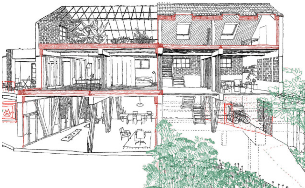
fig. 63 : Coupe perspective
