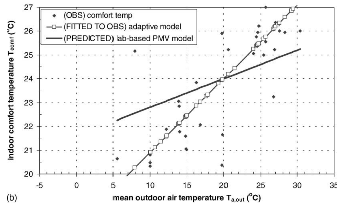
fig. 33 : Températures de confort intérieure observées et prévues pour les bâtiments climatisés (a) et pour les bâtiments à ventilation naturelle (b).
