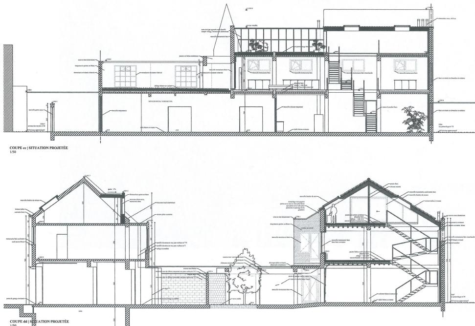
fig. 61 : Coupes (permis d'urbanisme)
