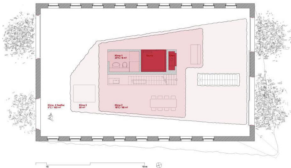
fig. 83 : Plan niv. +2
