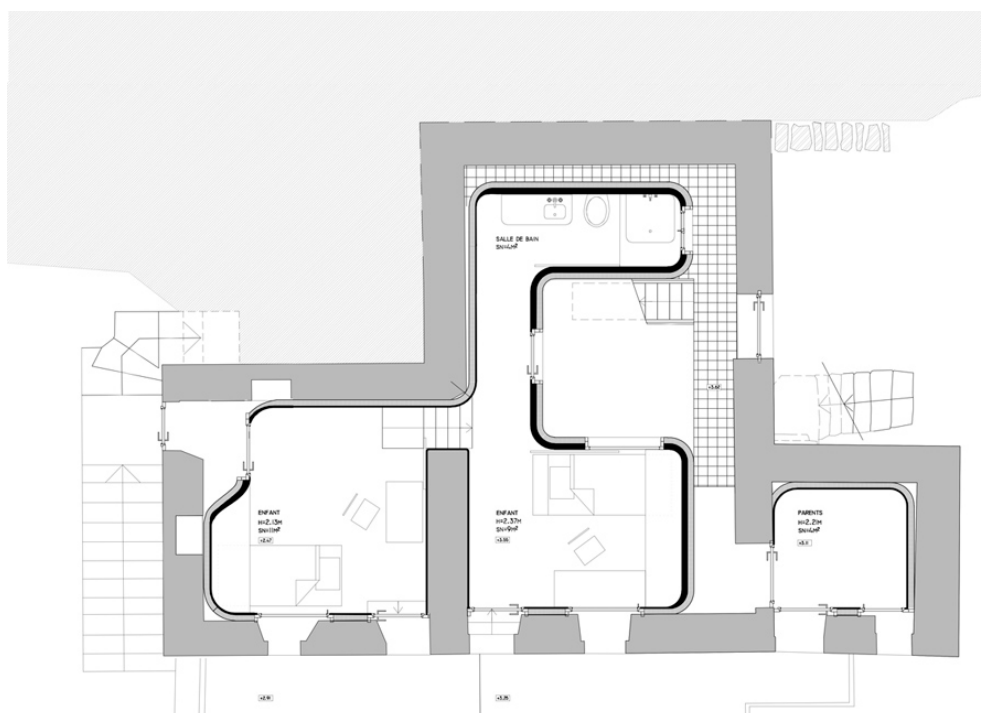
fig. 81 : Plan niv. +1
