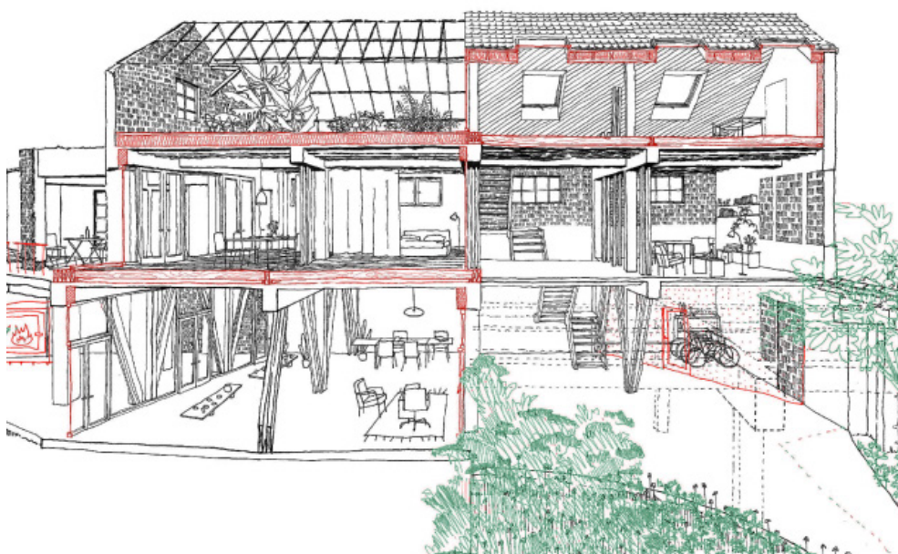
fig. 1 : Coupe perspective
