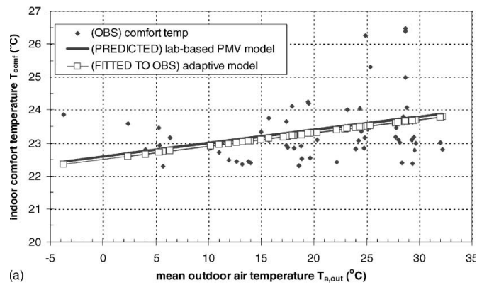
fig. 32 : Proposition de modèle de confort adaptatif de Richard J. de Dear et Gail S. Brager
