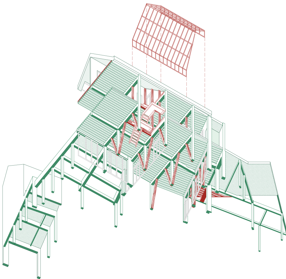
fig. 73 : axonométrie structurelle renversée
