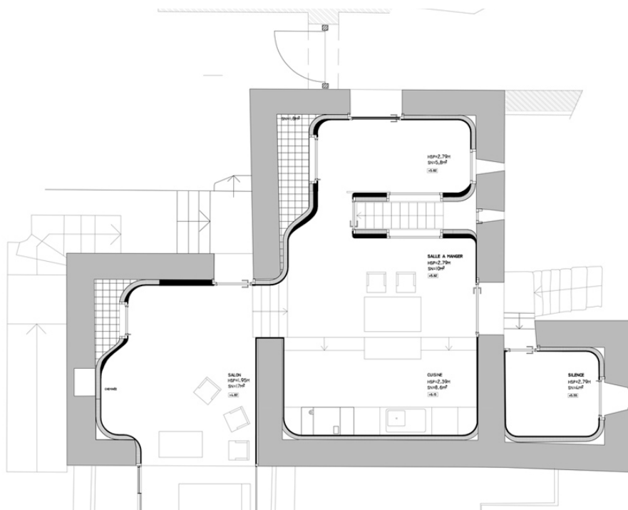
fig. 80 : Plan niv. +2
