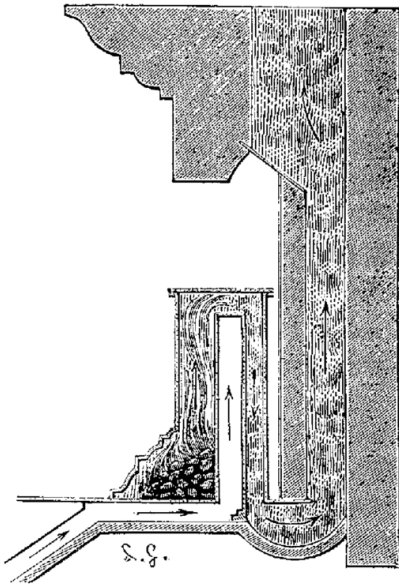
fig. 3 : Représentation du poêle Franklin
