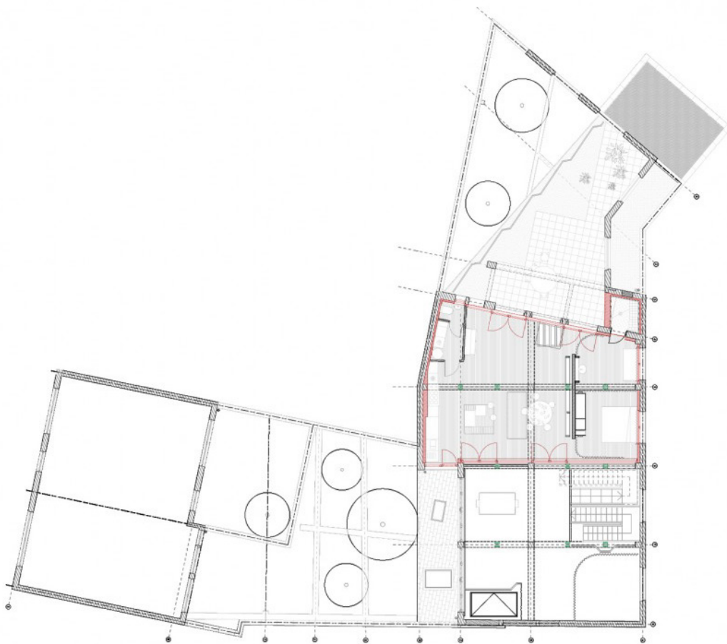
fig. 69 : Plan niv. +1
