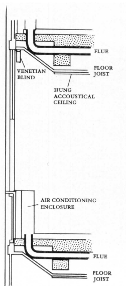
fig. 11 : Détail technique
