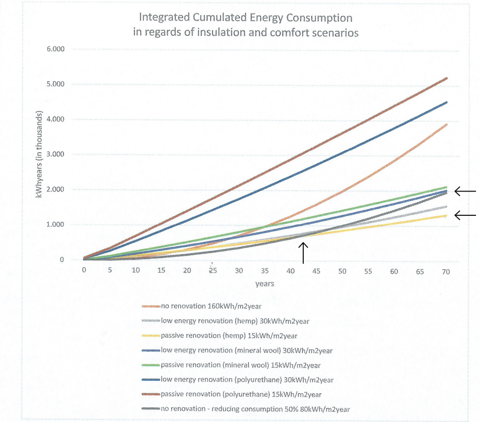
fig. 62 : Fiche de calcul comparant les différentes options
